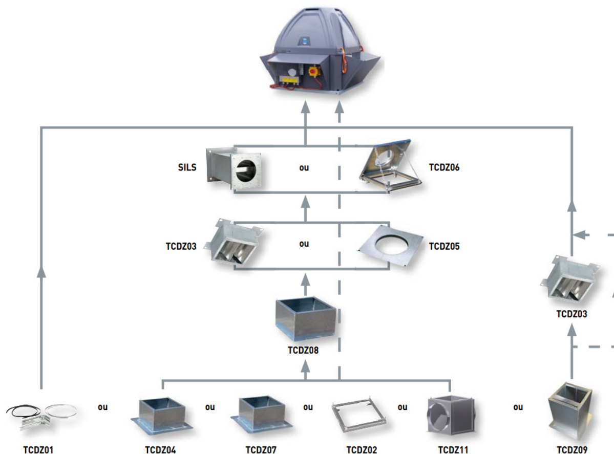
TEDH ECOWATT® / TEDV ECOWATT®
